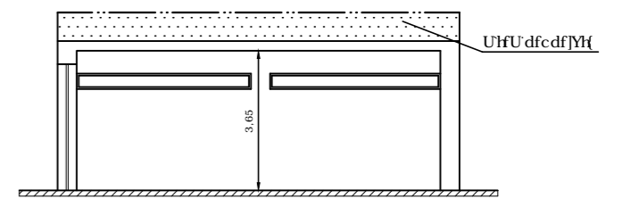
SEZIONE A-A
